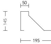
Abschnitt Dachhaltung
