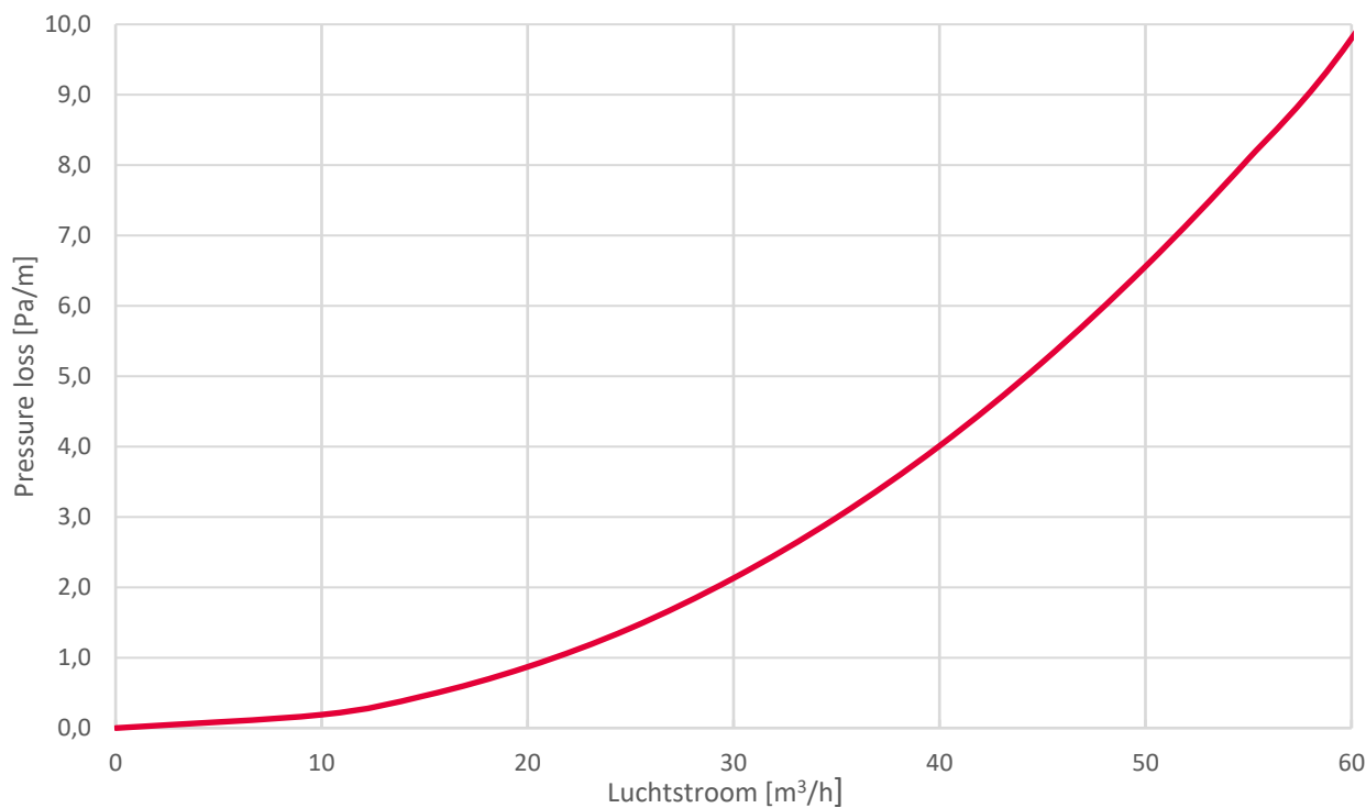
Drukverlies - flexibele ventilatiebuis 75 HEATPEX ARIA
