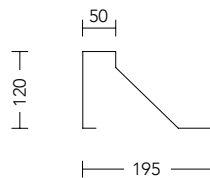
doorsnede
